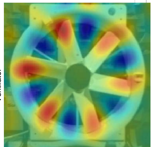
Ventilator
